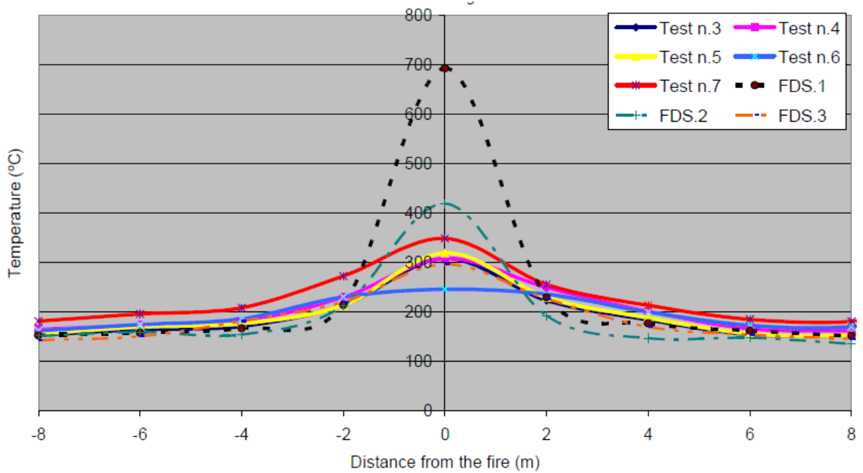
Temperature all'altezza del soffitto a 120 s per i 5 test e i 3 scenari di FDS
