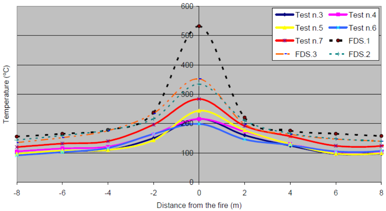
Temperature all'altezza del soffitto a 60 s per i 5 test e i 3 scenari di FDS
