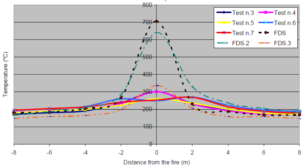
Temperature all'altezza del soffitto a 180 s per i 5 test e i 3 scenari di FDS
