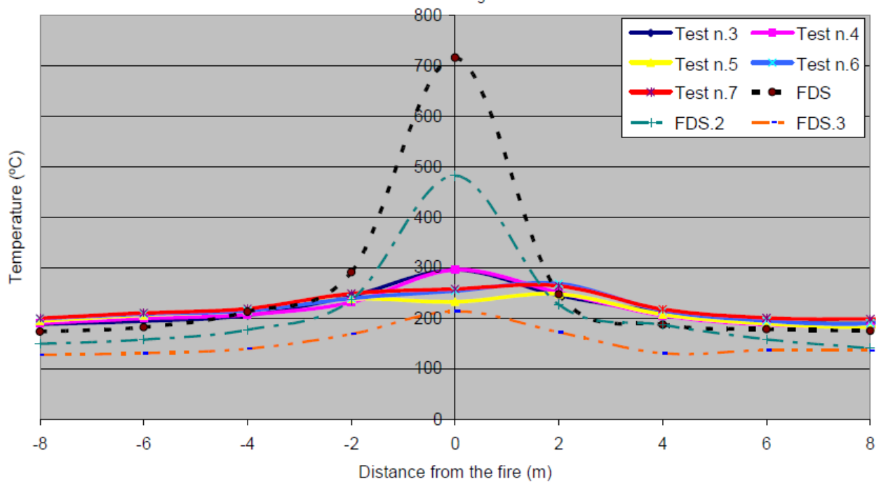
Temperature all'altezza del soffitto a 300 s per i 5 test e i 3 scenari di FDS
