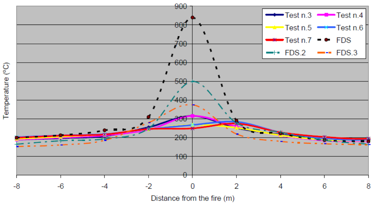
Temperature all'altezza del soffitto a 240 s per i 5 test e i 3 scenari di FDS
