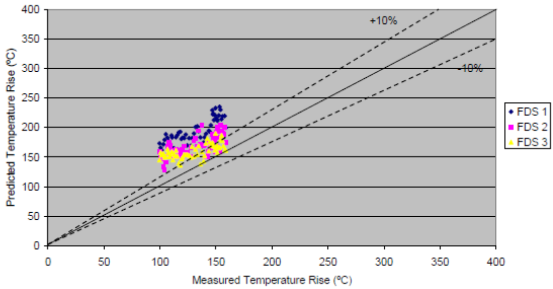
Valori calcolati da FDS confrontati con i valori previsti della temperatura dei gas (° C) tra 120s e 240s dall'accensione a una distanza di 6m del fuoco nella direzione del vento
