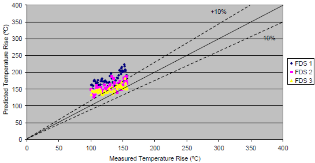
Valori calcolati da FDS confrontati con i valori previsti della temperatura dei gas (° C) tra 120s e 240s dall'accensione a una distanza di 8m del fuoco nella direzione del vento
