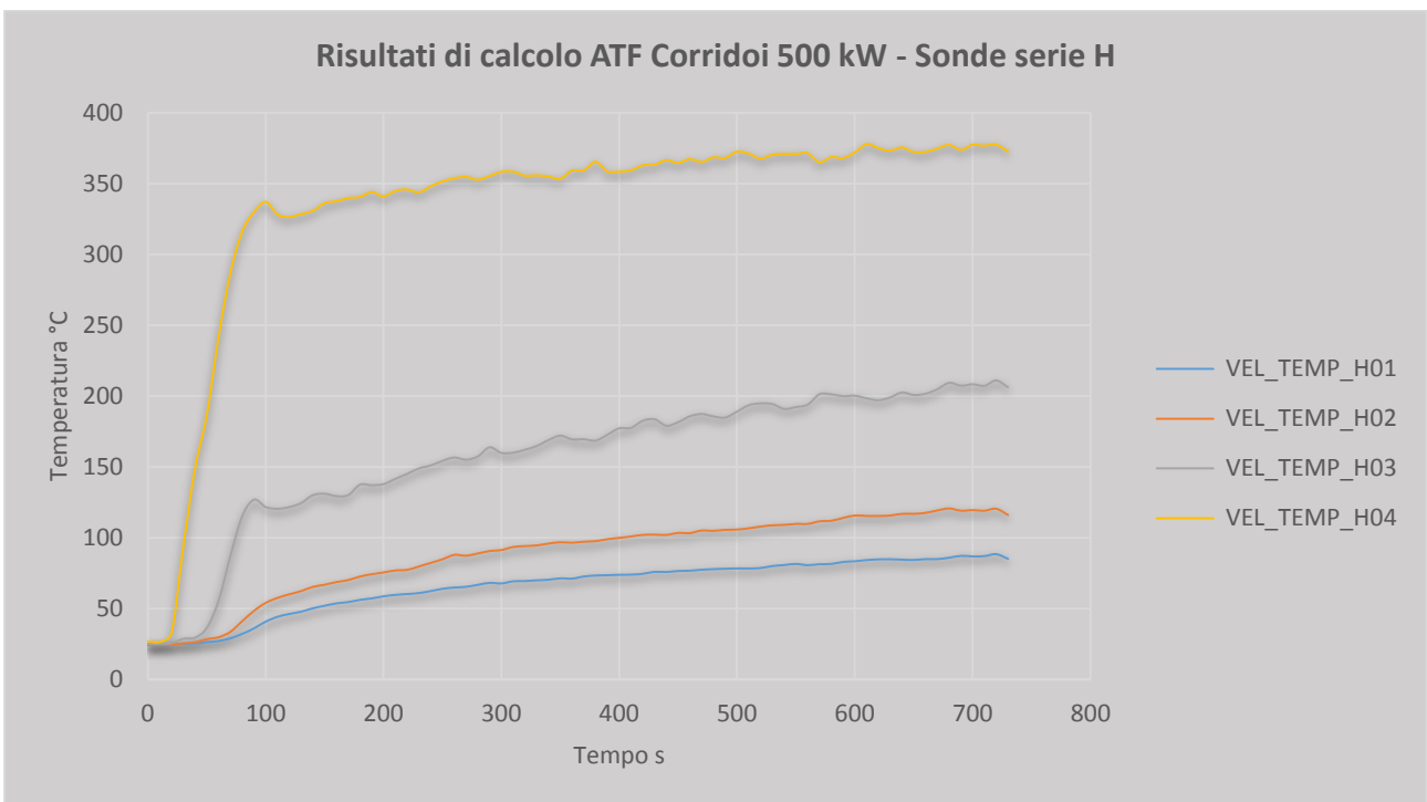
Risultati di calcolo e misurati per la serie di sonde di tipo H
