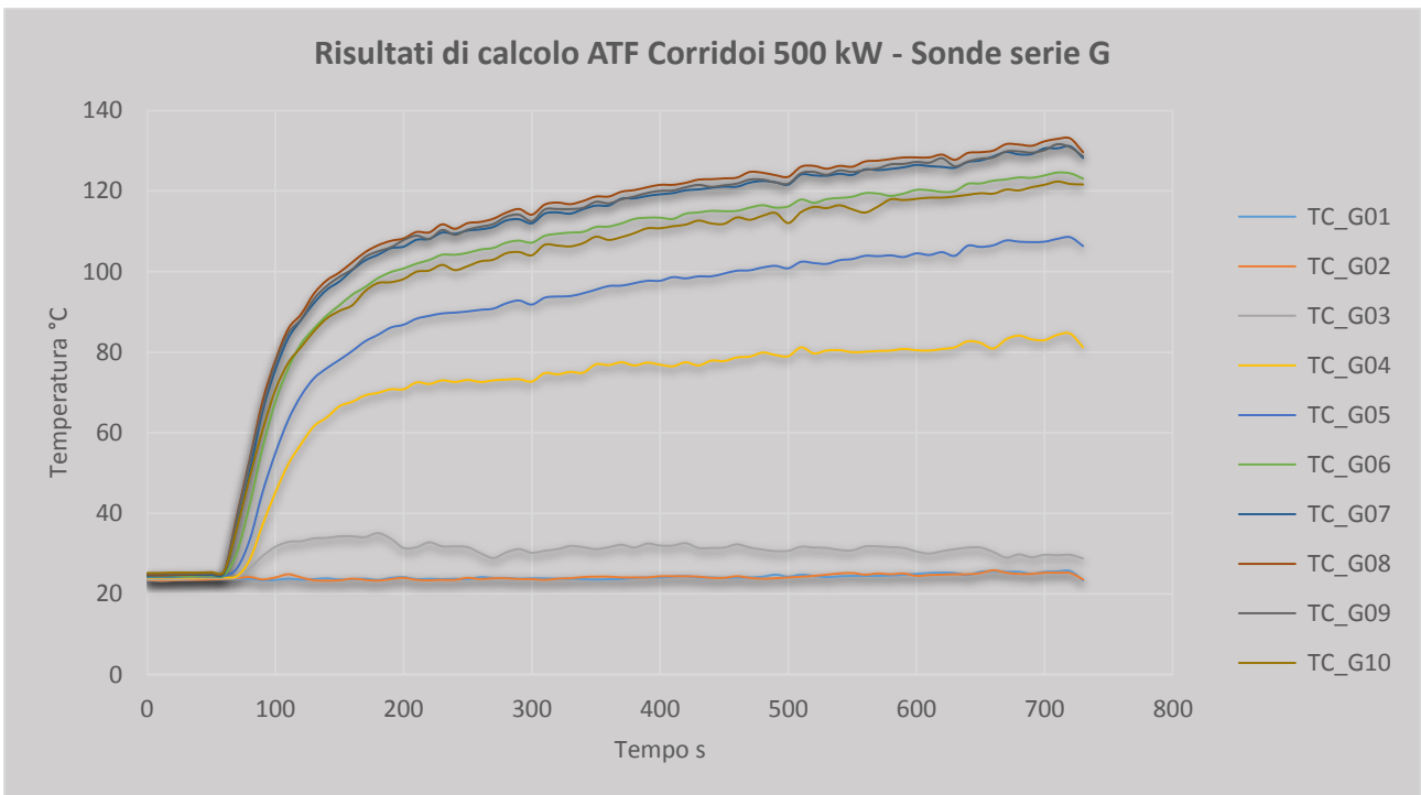
Risultati di calcolo e misurati per la serie di sonde di tipo G
