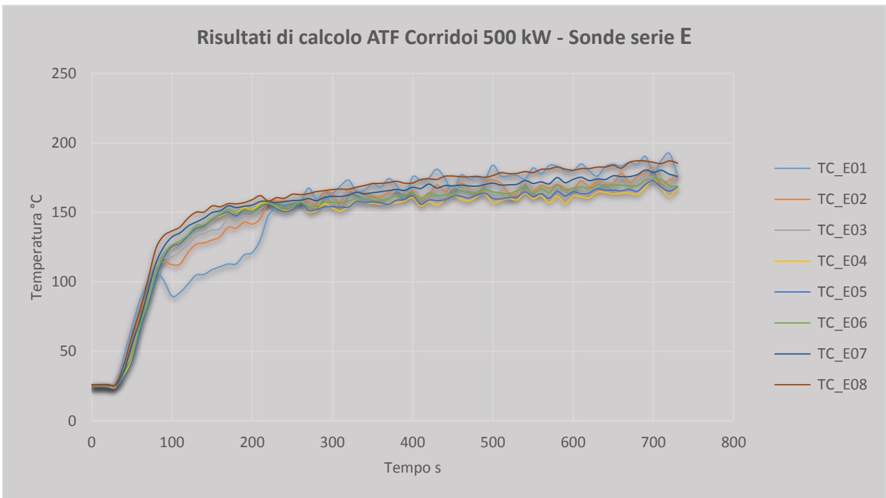
Risultati di calcolo e misurati per la serie di sonde di tipo E
